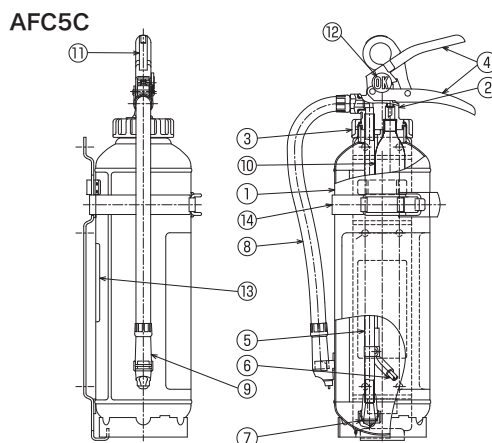
①本体容器 ②上部金具 ③キャップ ④レバー ⑤サイホン管 ⑥ガス導入管 ⑦粉上り防止封板 ⑧ホース ⑨ノズル ⑩加圧用ガス容器 ⑪安全栓 ⑫OKマーク ⑬リサイクルシール ⑭プラケット
