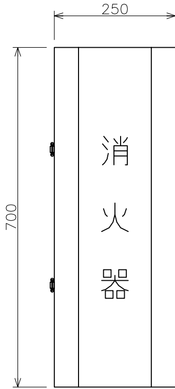
正面図
