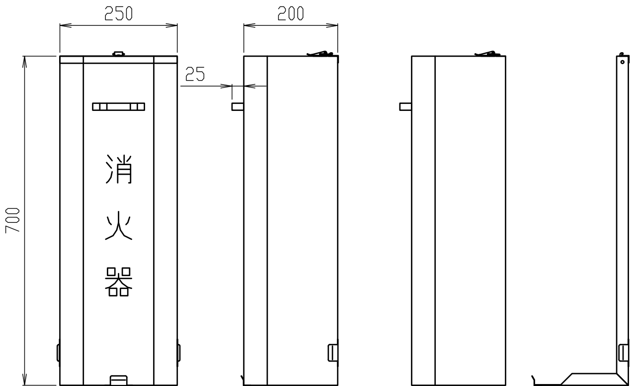
正面図
