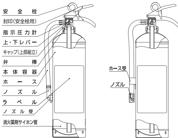
上図は代表消火器の事例です。機種により形状・構造が異なるものがあります。
