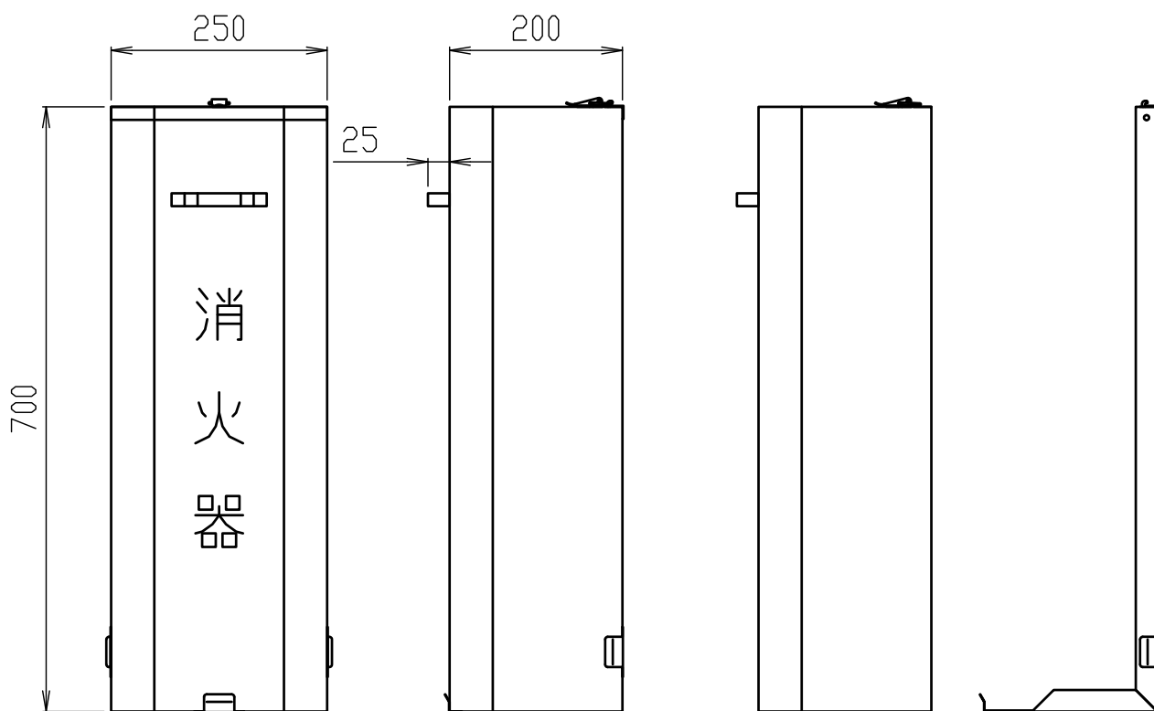
正面図
